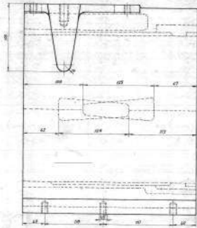
A-A Kesiti
